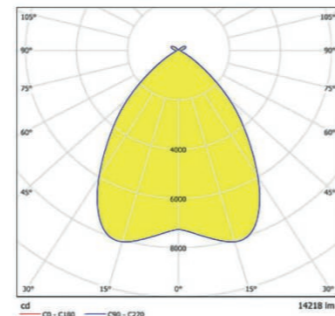
Проект осветительной установки на базе МГЛ-светильника ГСП17-250 с лампой OSRAM POWERSTAR HQI-E 250W
