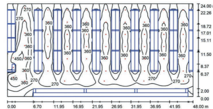
#2. Проект осветительной установки на базе LED-светильника LED UniLED 80W-LUX-PR
