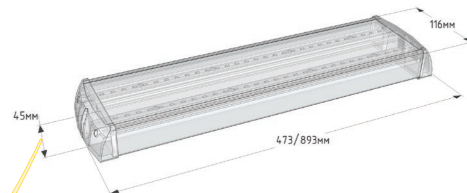
Габаритный чертеж светильника
