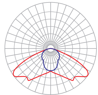
Кривая силы света (КСС)
