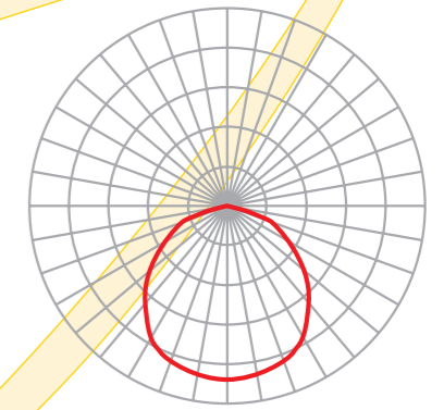
Кривая силы света 120 град (KCS)
