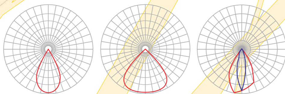
Кривые силы света (КСС)
