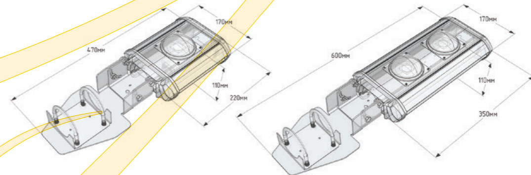
Габаритный чертеж
