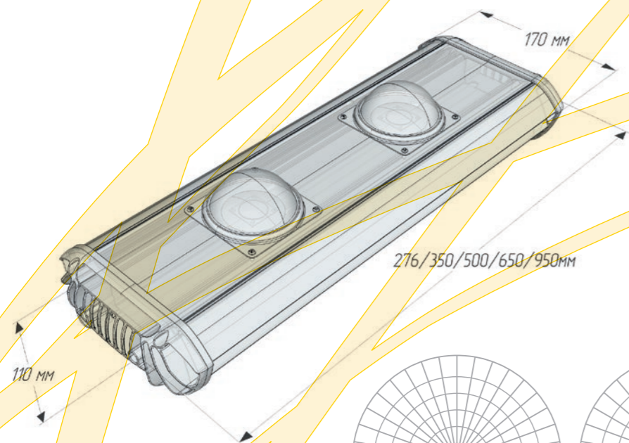
Габаритный чертеж
