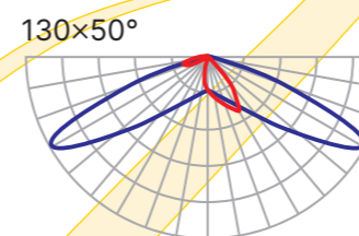
Кривые силы света (КСС)
