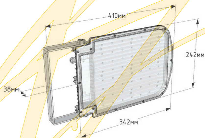
Габаритный чертеж
