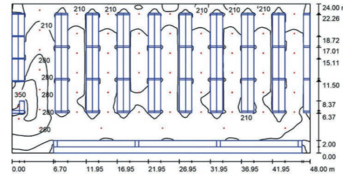
#1. Проект осветительной установки на базе LED-светильника LED UniLED ECO-MP 100W60x20
