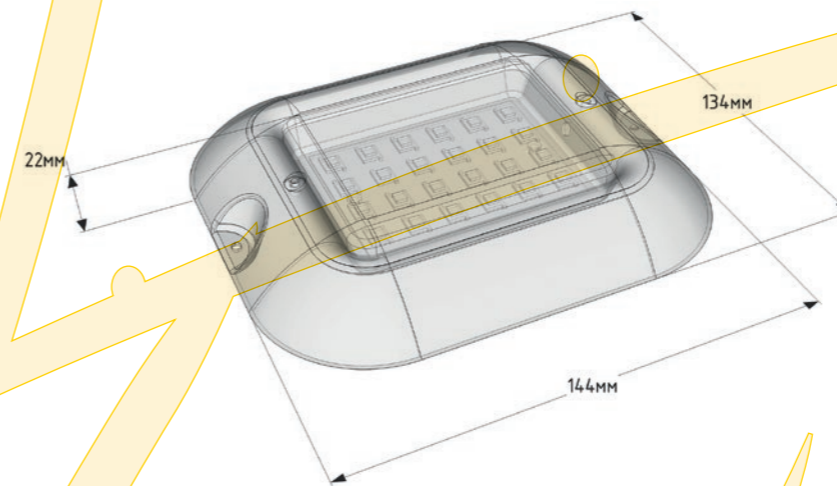
Габаритный чертеж
