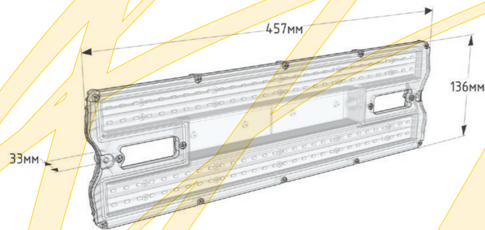
Габаритный чертеж
