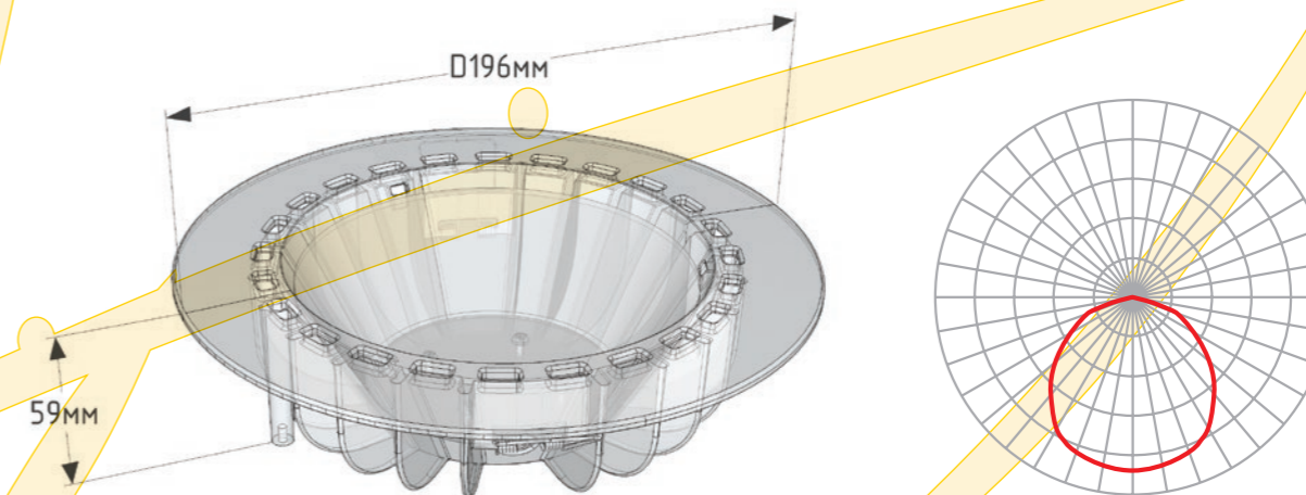
Габаритный чертеж
