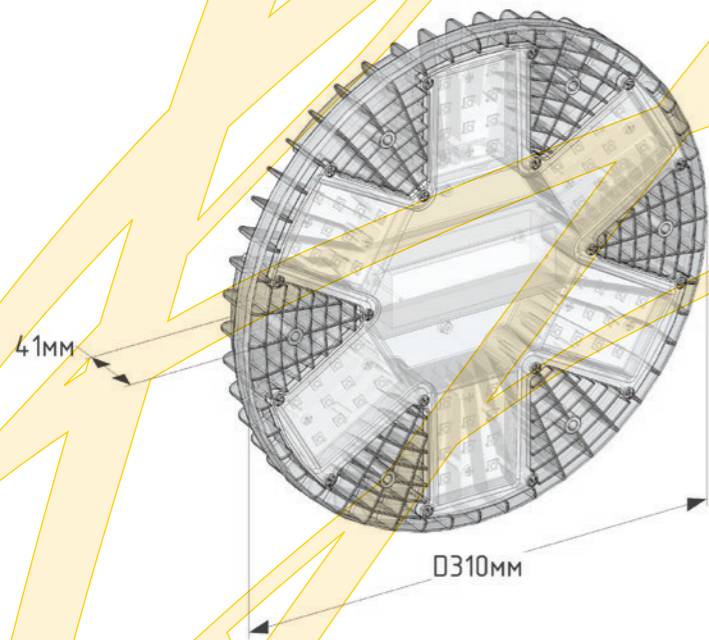
Габаритный чертеж
