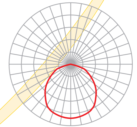
Кривая силы света 120 град (KCC)
